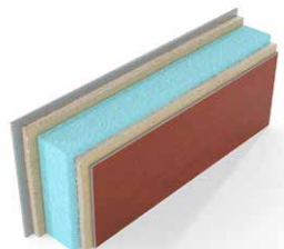
MIXTO 26 MM MADERA 4 + 4 MM POLIESTIRENO 18 MM
